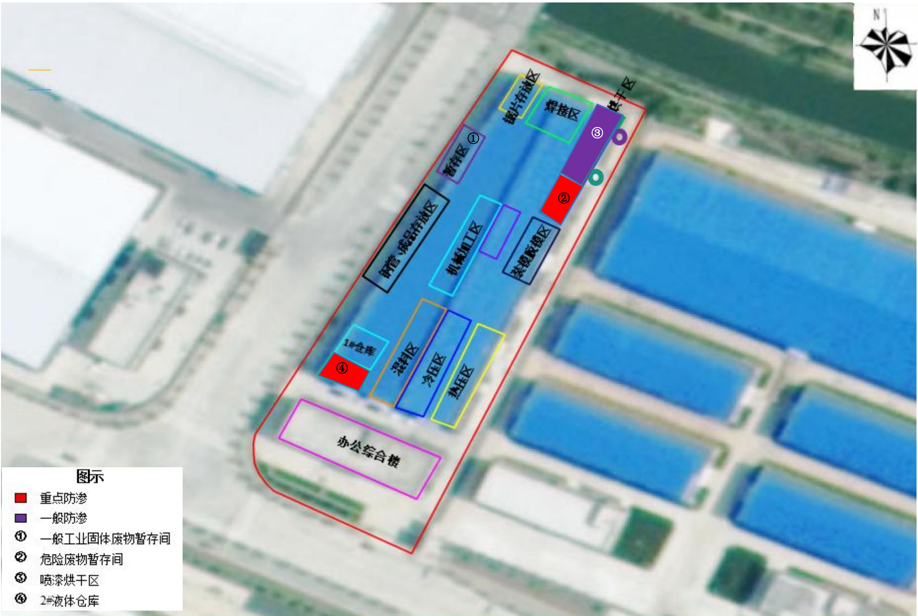
附图6 项目分区防渗图
